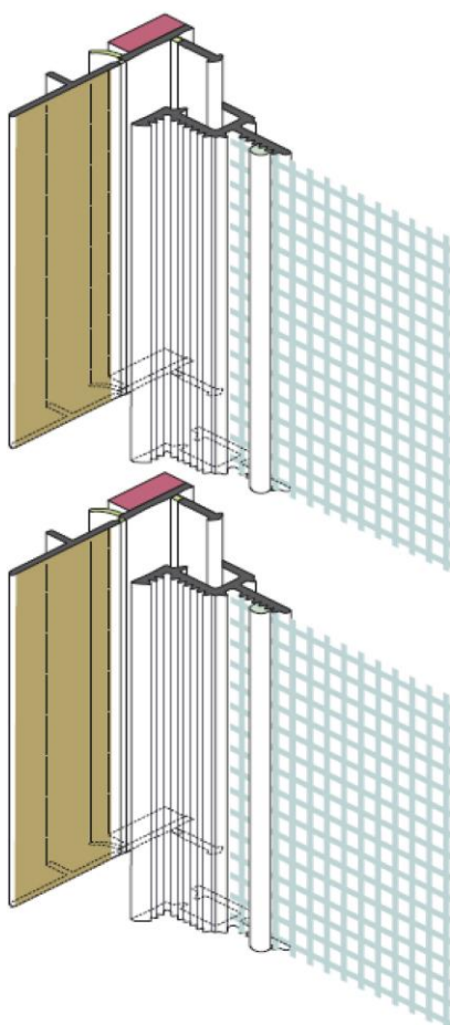
Abbildung 3: Stoßausbildung
