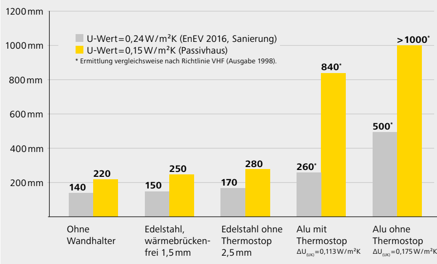
Erforderliche Dämmstoffdicken unter Berücksichtigung von Wärmebrücken durch metallische Unterkonstruktion für bestimmte U-Werte.
