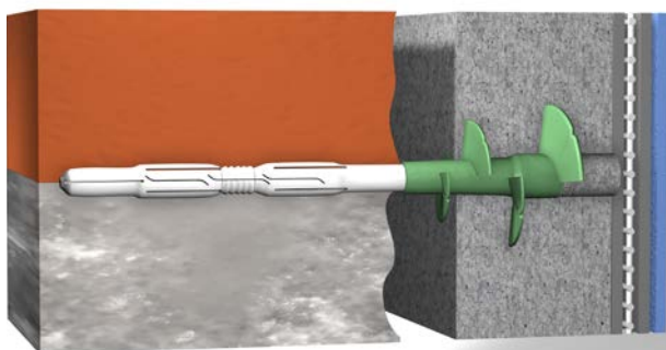
Optimal aufeinander abgestimmte Systemkomponenten ermöglichen die sichere Verankerung und exakte Justierbarkeit des WDV-Systems.
